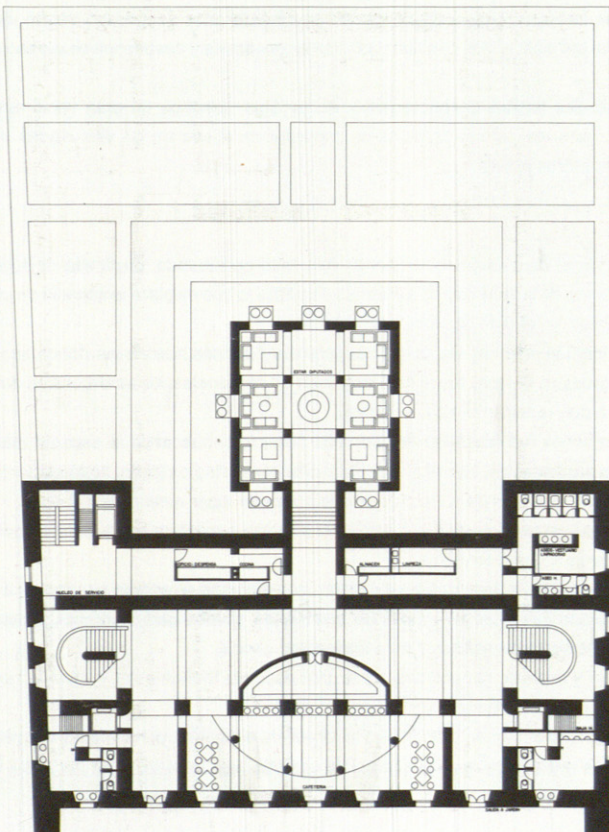
Planta sótano.
