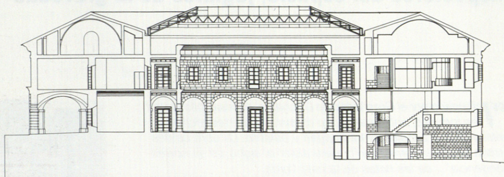
Sección Este-Oeste.
