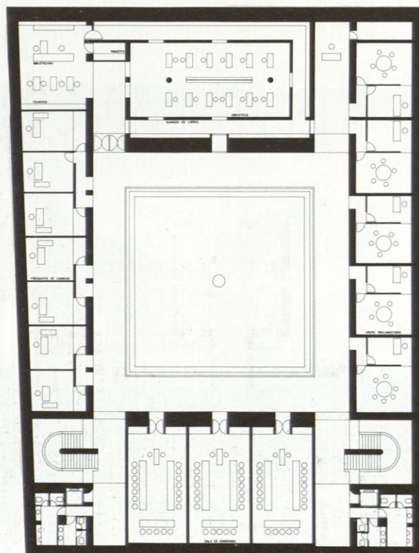
Planta tercera.
