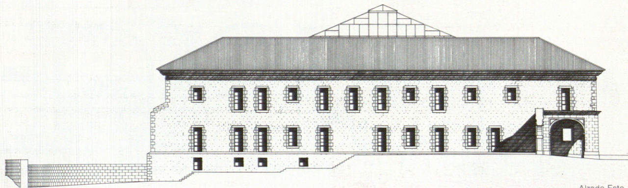
Alzado Este.
